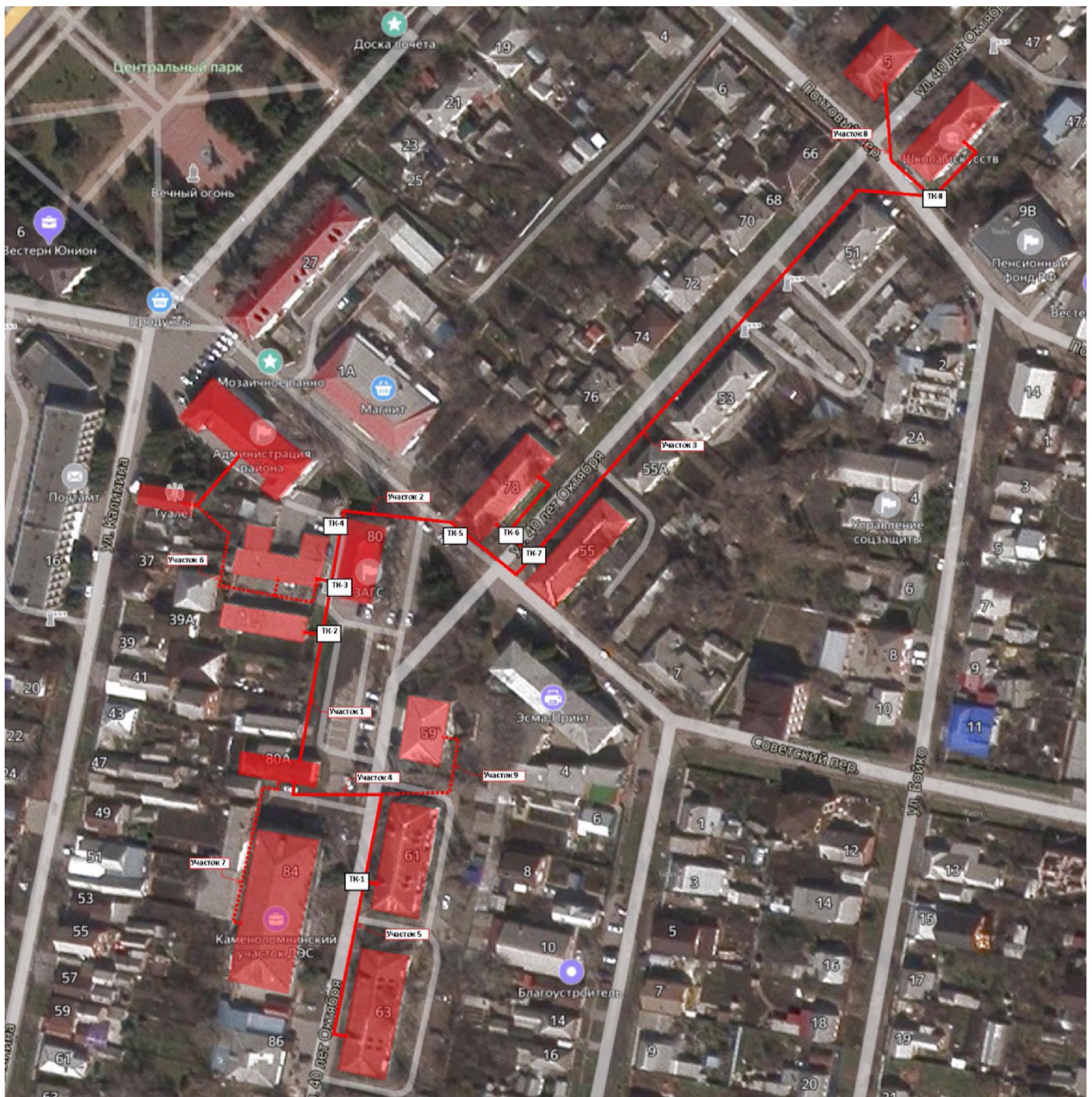
Рис. 4 – Схема тепловых сетей от котельной ул. 40 лет Октября 80а
